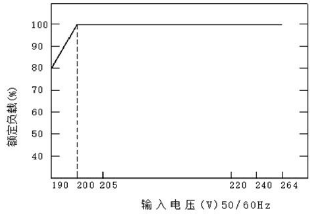
输入电压与负载曲线
