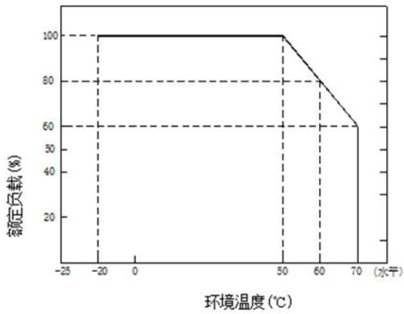
输出负载与温度曲线
